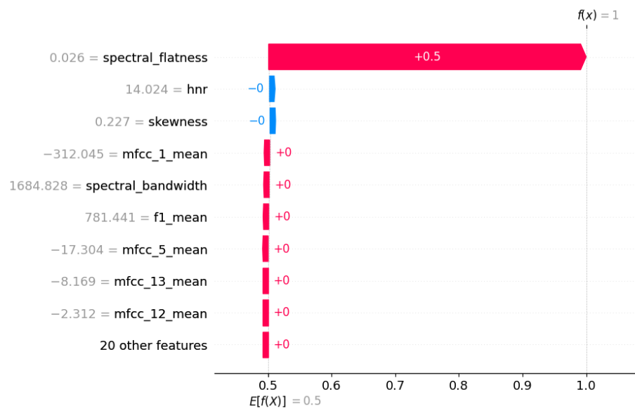
Figura 39: Explicación local con SHAP
