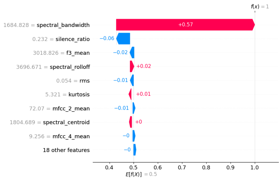
Figura 44: Explicación local con SHAP tras quitar spectral flatness y mfcc 1
