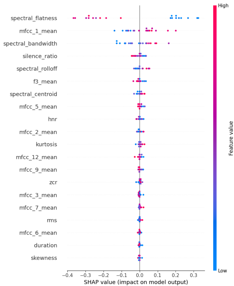
Figura 32: Explicación global con SHAP
