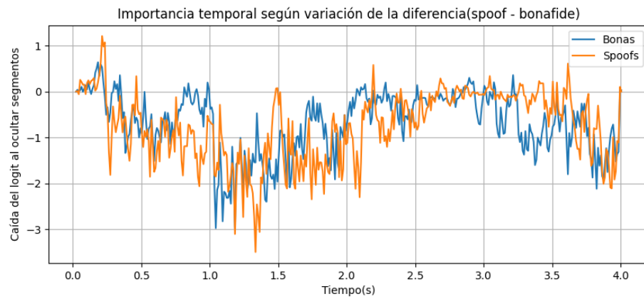
Figura 56: Resultados de margen de la ocultación temporal en AASIST.
