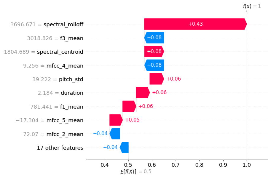
Figura 51: Explicación local con SHAP tras quitar spectral flatness, mfcc 1 y spectral bandwidth
