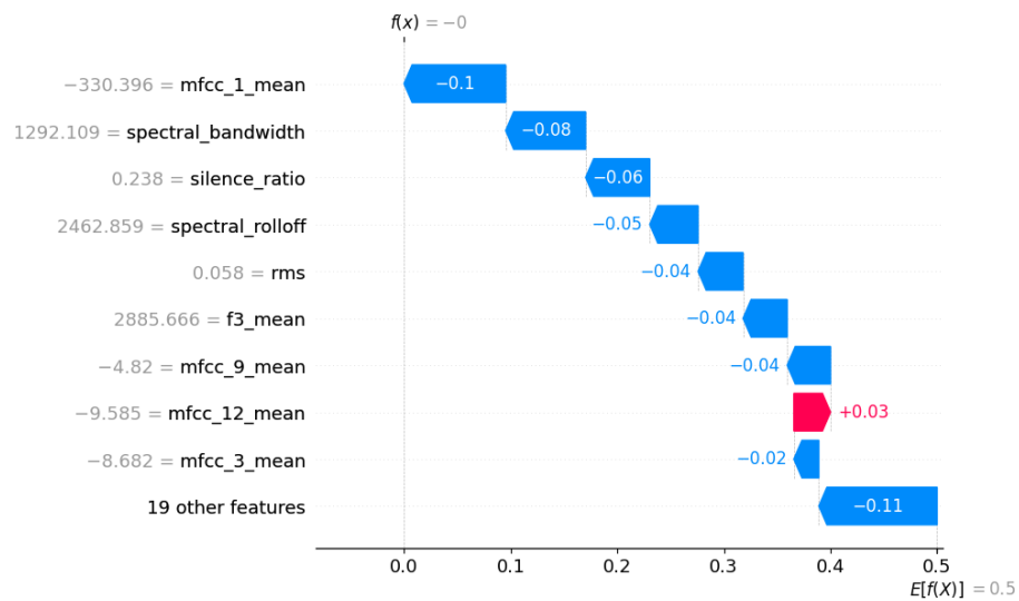
Figura 48: Explicación local con SHAP tras quitar spectral flatness
