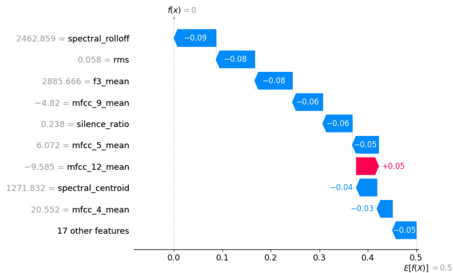
Figura 50: Explicación local con SHAP tras quitar spectral flatness, mfcc 1 y spectral bandwidth
