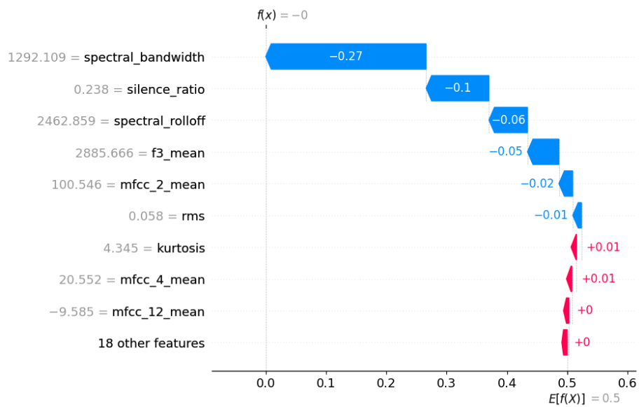
Figura 43: Explicación local con SHAP tras quitar spectral flatness y mfcc 1
