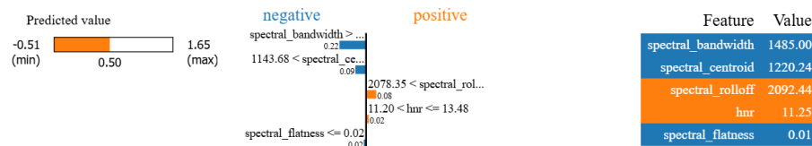
Figura 14: Explicación local espectrales Lime.
