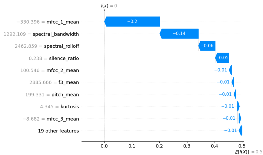
Figura 33: Explicación local con SHAP tras quitar spectral flatness
