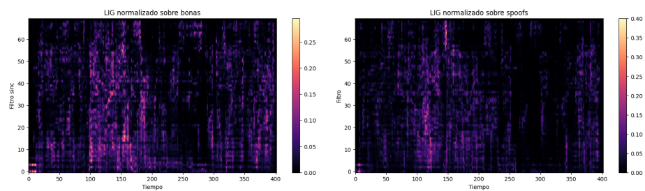
(a) Mapa filtro-tiempo normalizado generado con IG para “bonas”. (b) Mapa filtro-tiempo normalizado generado con IG para “spoofs”.
