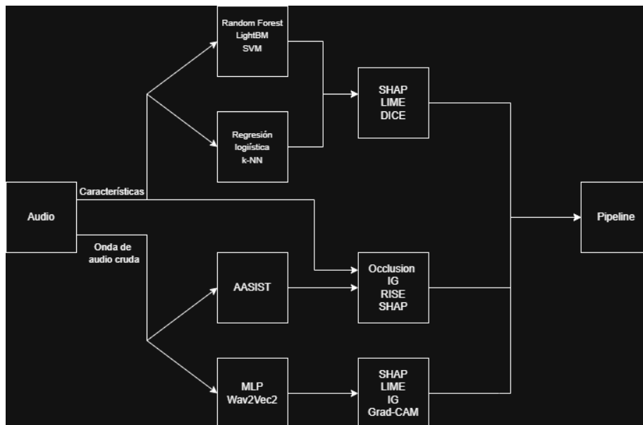
Figura 54: Arquitectura del pipeline.
