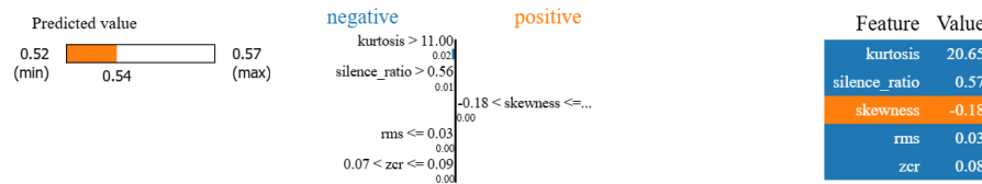
Figura 13: Explicación local energía Lime.
