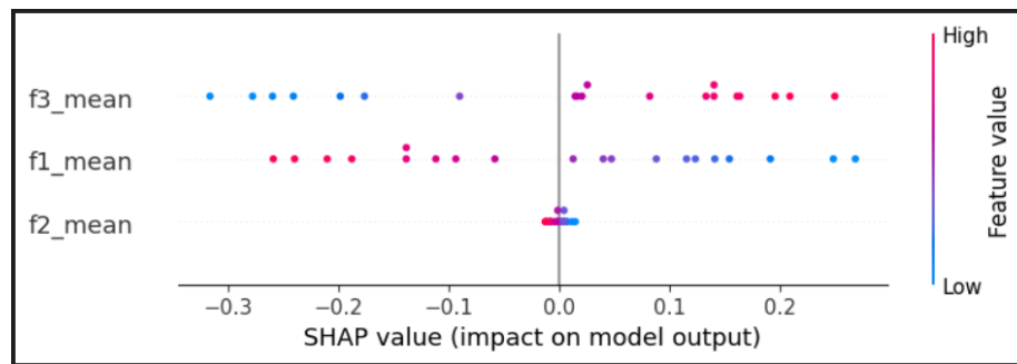
Figura 9: Shap global formantes.
