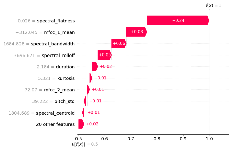
Figura 31: Explicación local con SHAP
