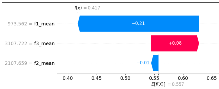
Figura 10: Ejemplo concreto (I_12_N).
