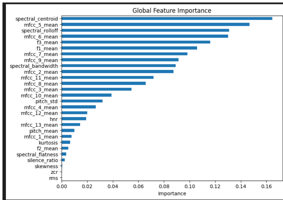
Figura 20: Ranking agregado de características.
