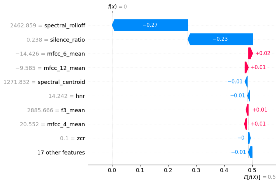
Figura 35: Explicación local con SHAP tras quitar spectral flatness, mfcc 1 y spectral bandwidth
