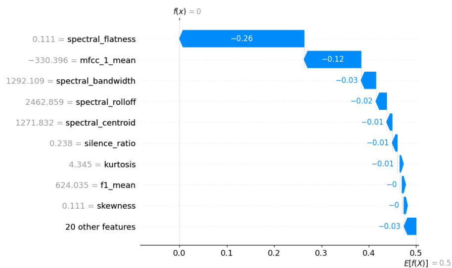
Figura 30: Explicación local con SHAP
