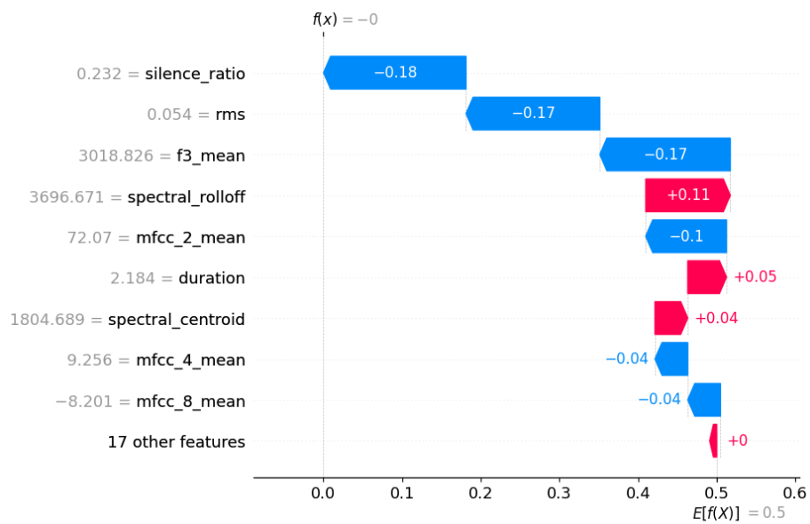
Figura 36: Explicación local con SHAP tras quitar spectral flatness, mfcc 1 y spectral bandwidth
