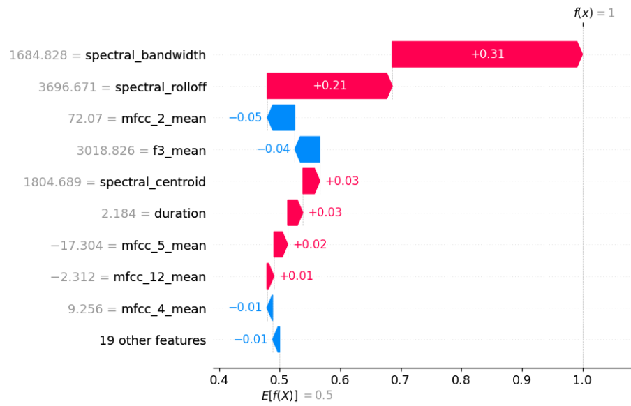
Figura 34: Explicación local con SHAP tras quitar spectral flatness
