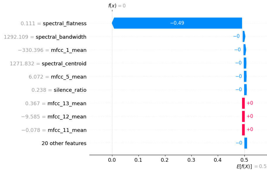
Figura 38: Explicación local con SHAP
