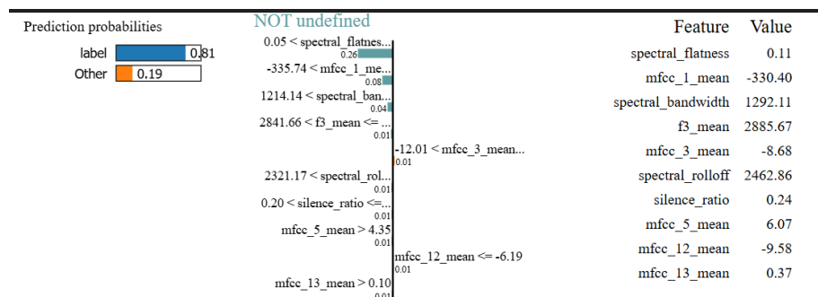
Figura 45: Explicación local con LIME
