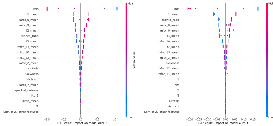
(a) Agrupación de las gráficas SHAP del clasificador.
