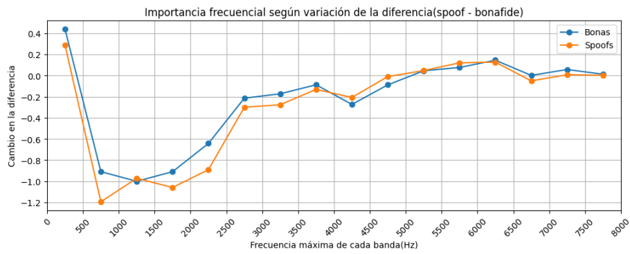
Figura 58: Resultados de margen de la ocultación frecuencial en AASIST.
