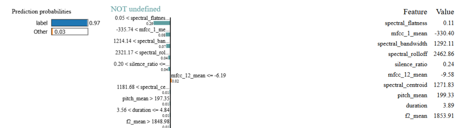
Figura 37: Explicación local con LIME
