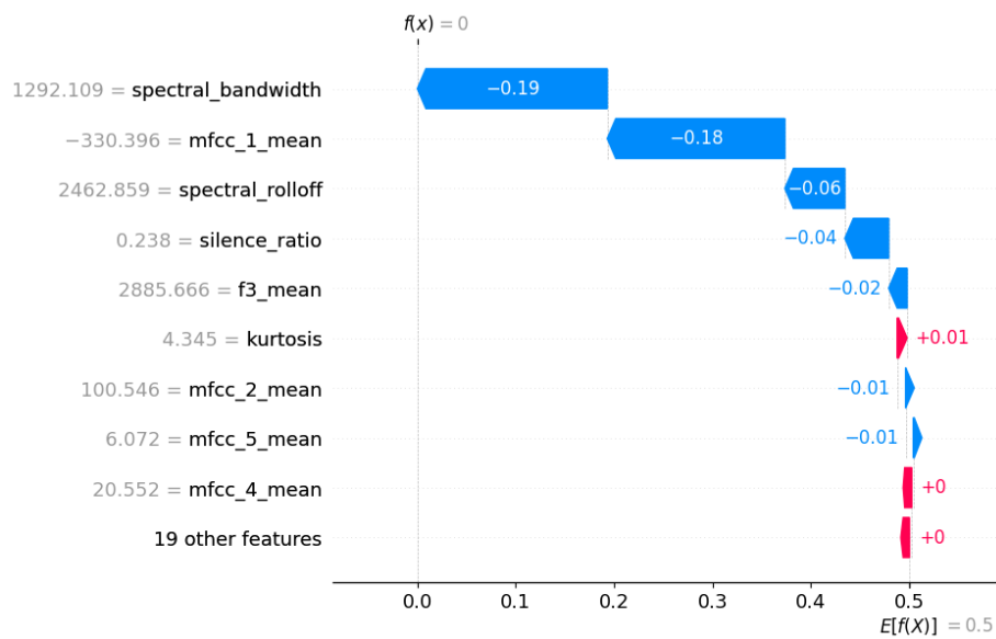
Figura 41: Explicación local con SHAP tras quitar spectral flatness
