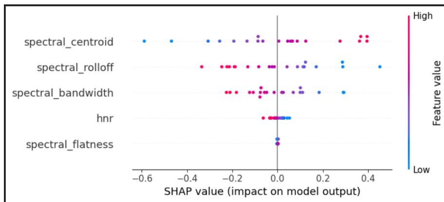
Figura 5: Shap global espectrales.
